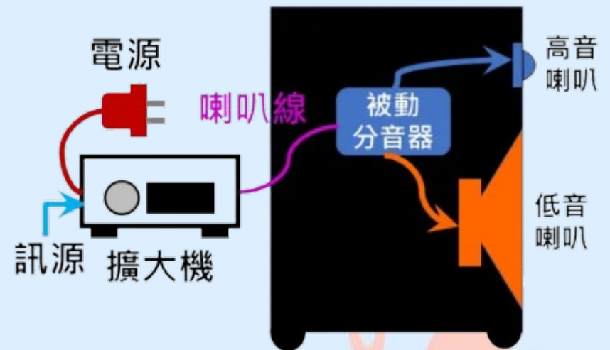
被動式喇叭
