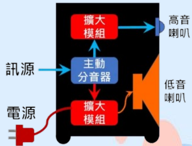
主動式喇叭
